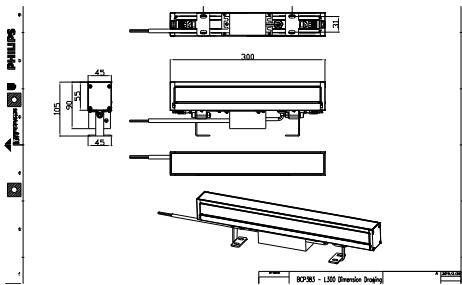
BCP383 9LED RGB 220V A2 L30 DMX D2
