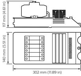
DMP603GL-CE
